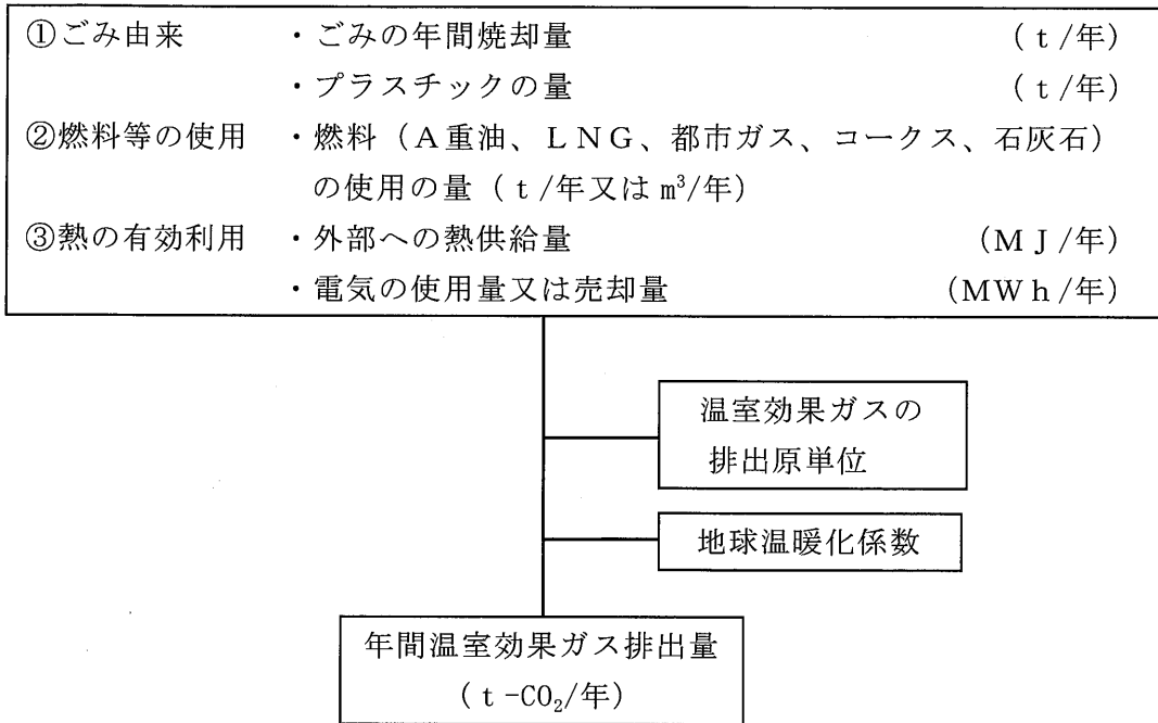
図 7-9-1-1 施設の稼働に伴う温室効果ガス排出量の算定手順
