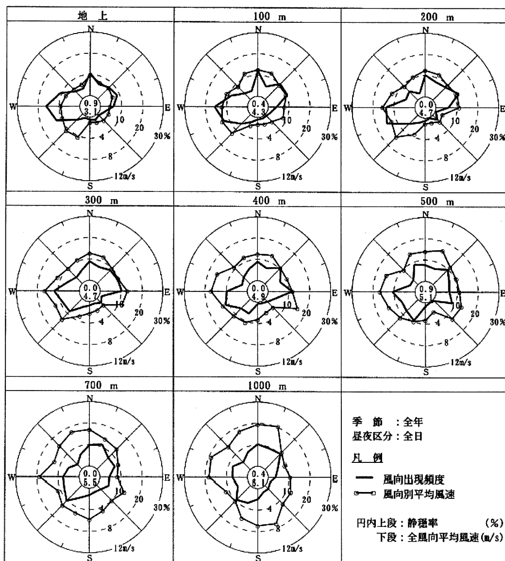
図 6-1-1-2 高度別風配図及び風向別平均風速
